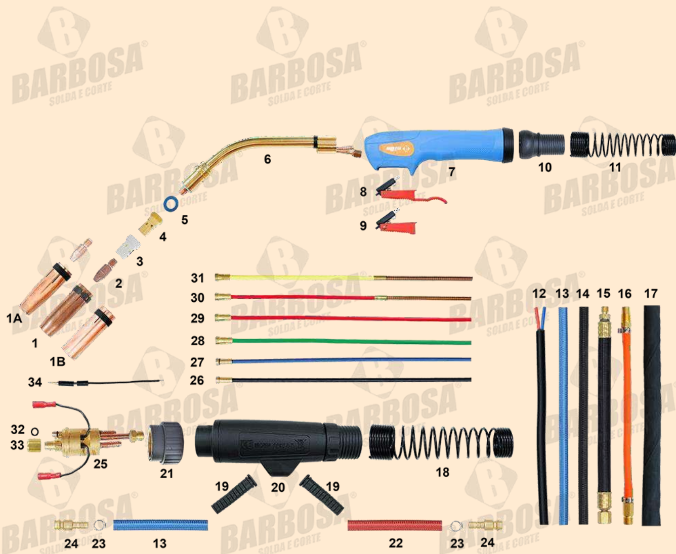
Tocha Ergo MIG/MAG 501W
