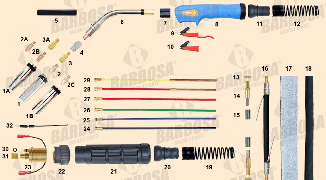
Tocha Ergo MIG/MAG 36
