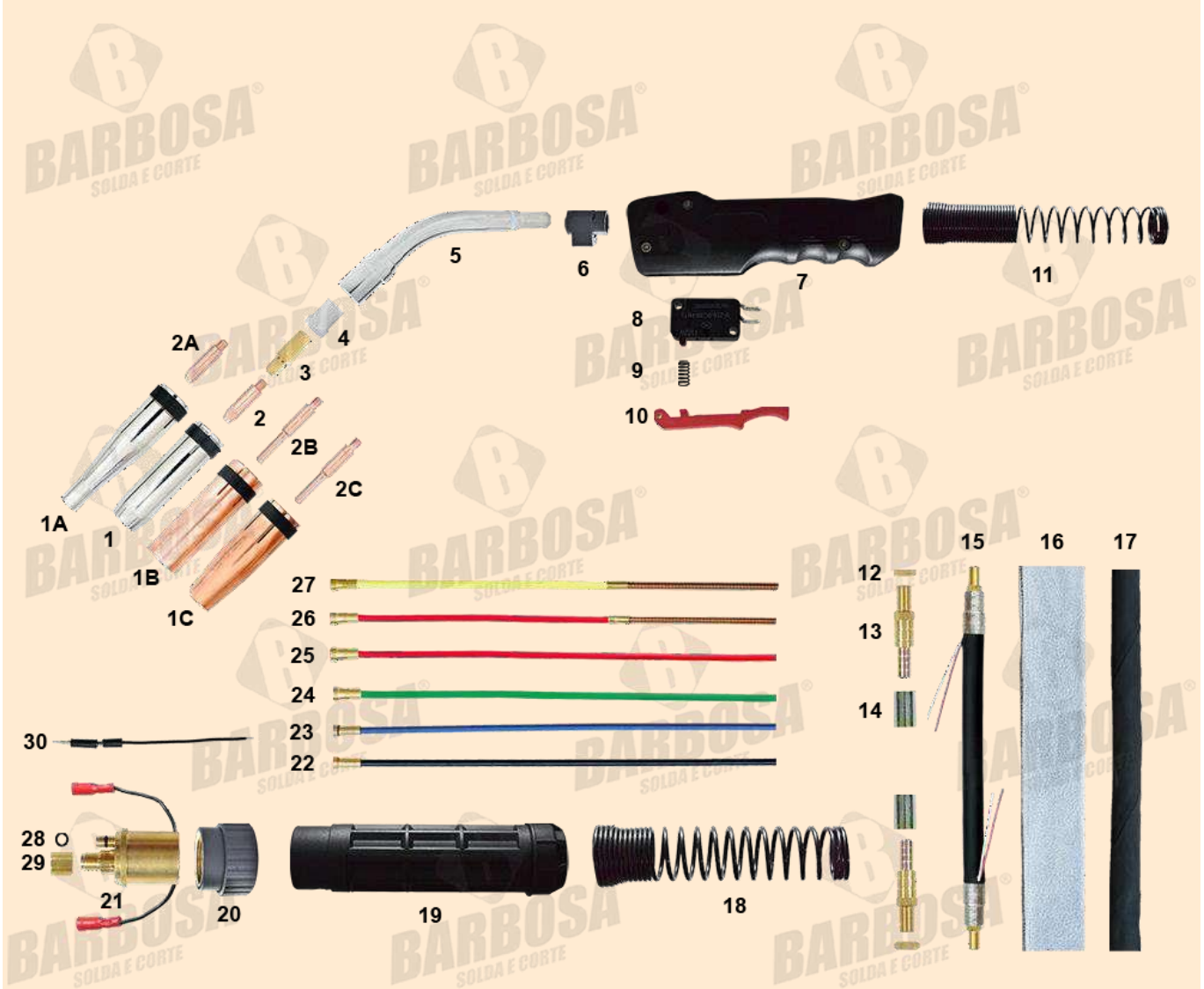
Tocha Ergo MIG/MAG 135
