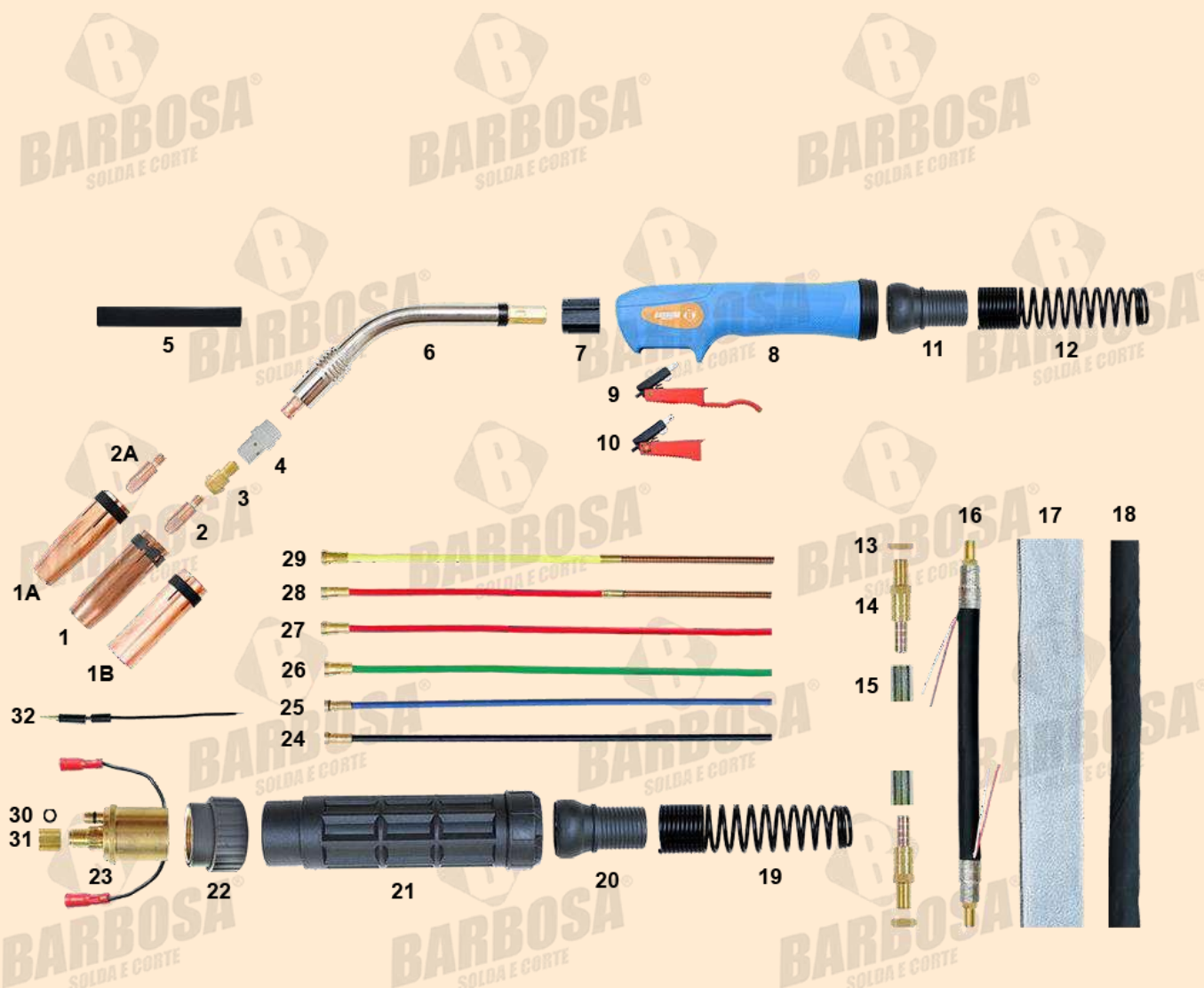
Tocha Ergo MIG/MAG 26
