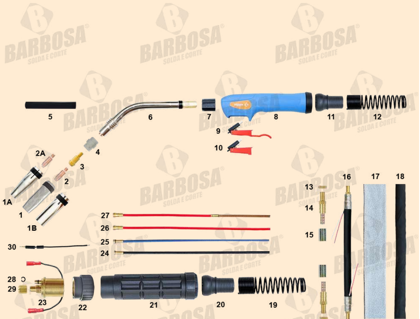
Tocha Ergo MIG/MAG 24
