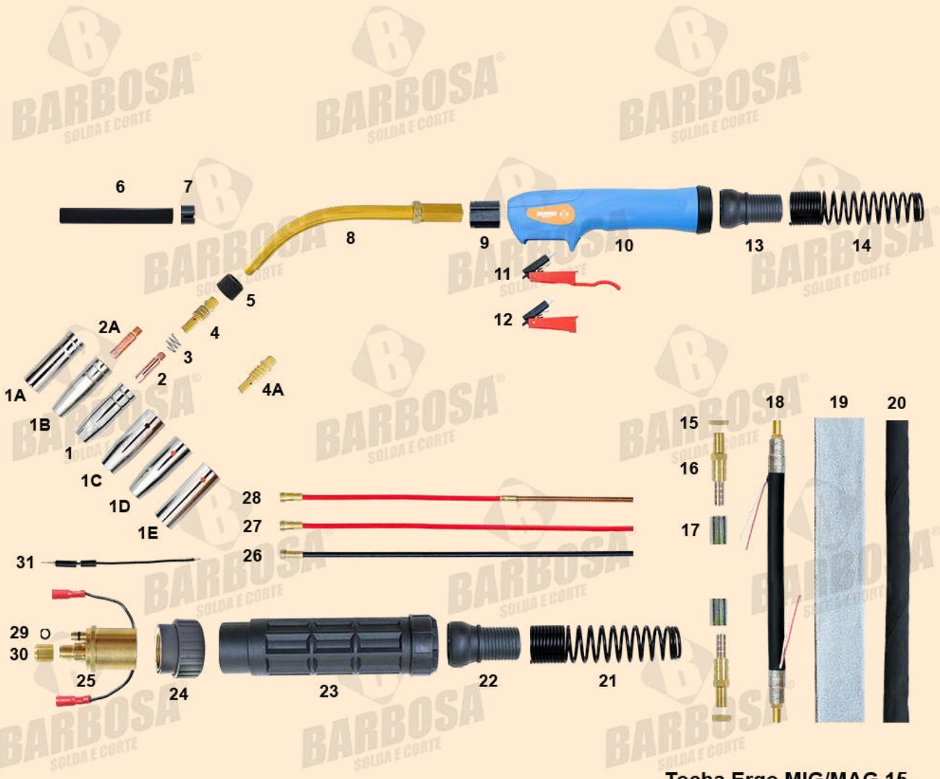
Tocha Ergo MIG/MAG 15
