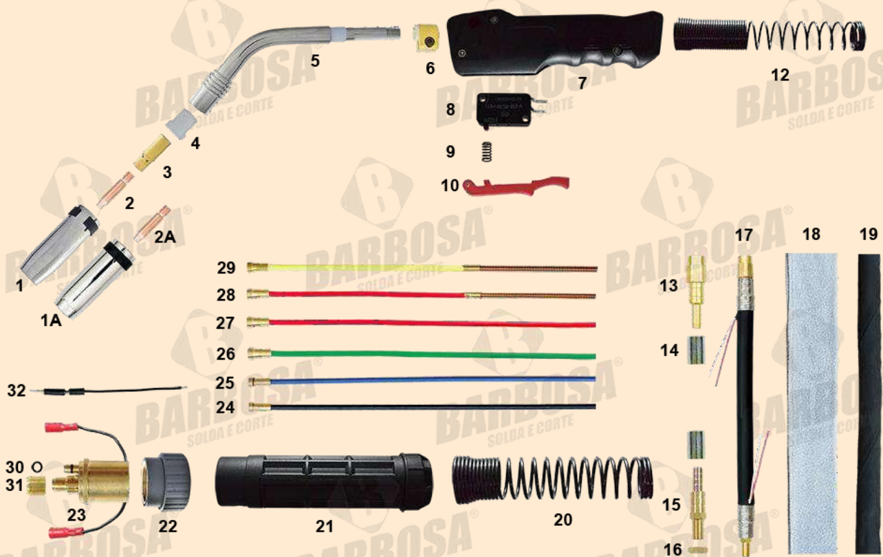
Tocha Ergo MIG/MAG 350
