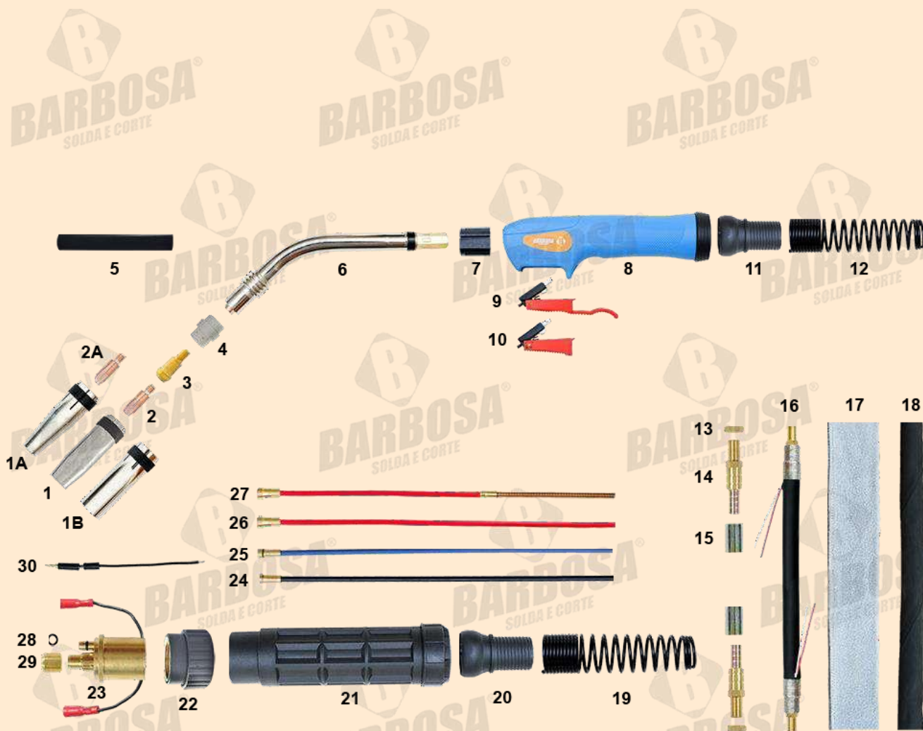
Tocha Ergo MIG/MAG 24
